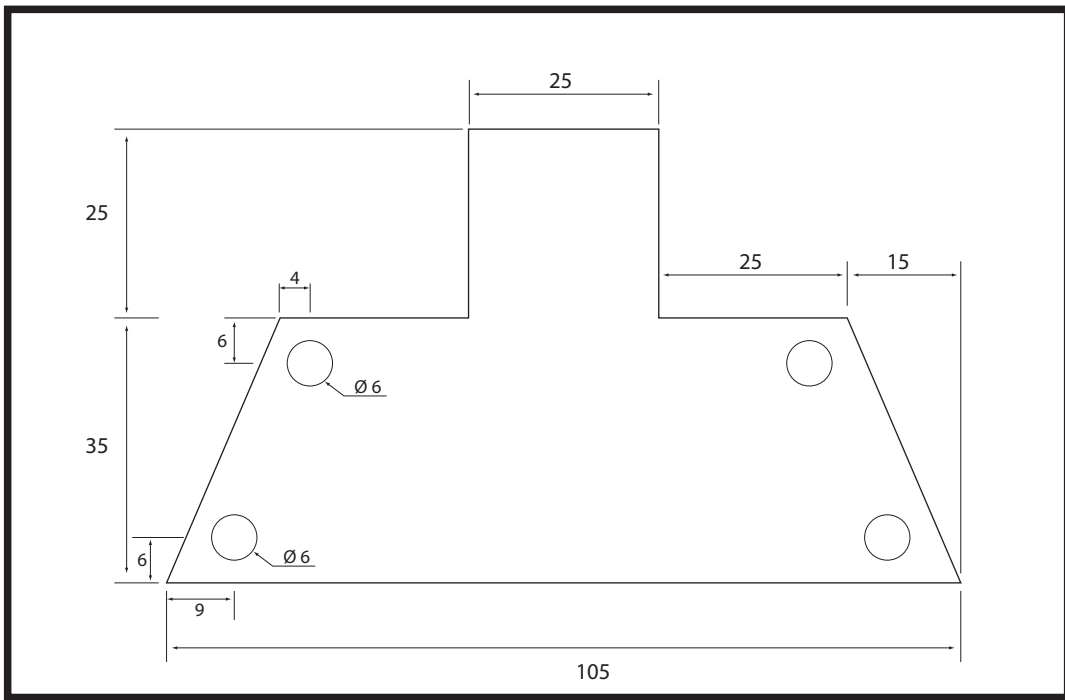
Flancs (x2)
